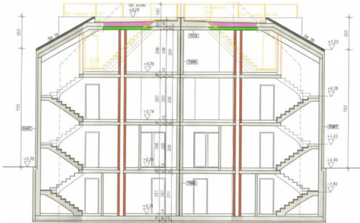
Schnitt B-B
