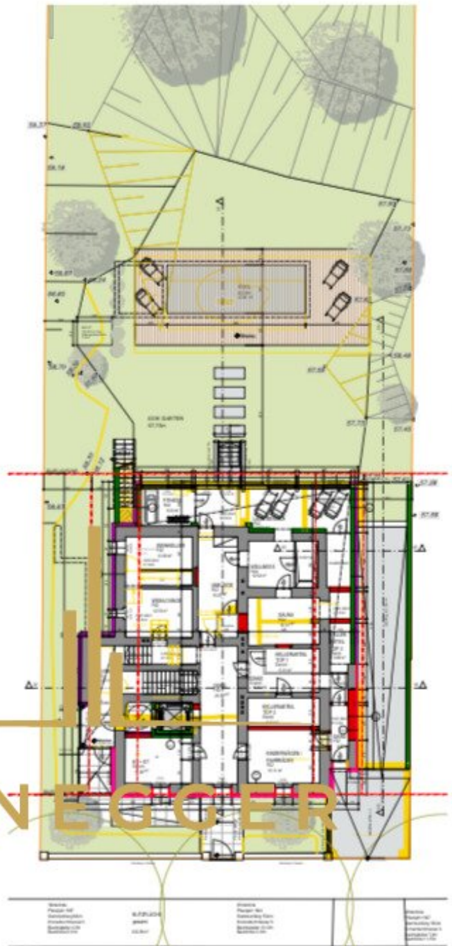
GRUNDRISS TIEFGESCHOSS (Baustufe 1, Konzept) M 1:100
