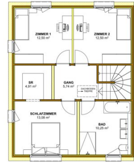
OBERGESCHOSS
