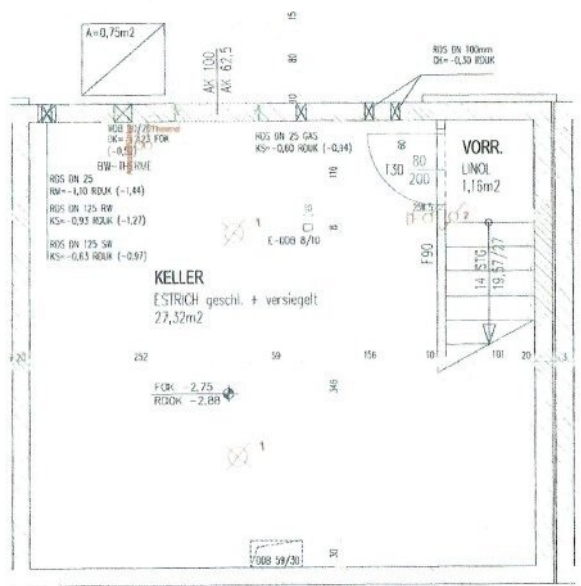
KELLERGESCHOSS
