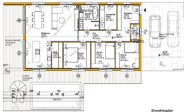
Grundrissplan
