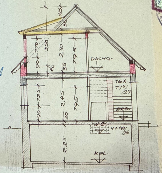
SCHNITT A-B
