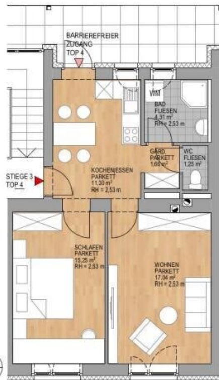
GRUNDRISS 1:100
