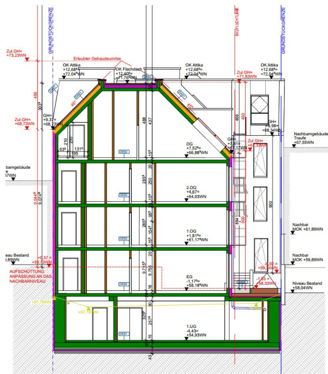
SCHNITT B-B 1:100
