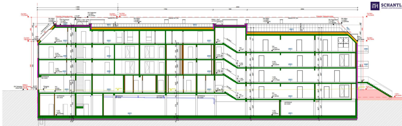
SCHNITT C-C
