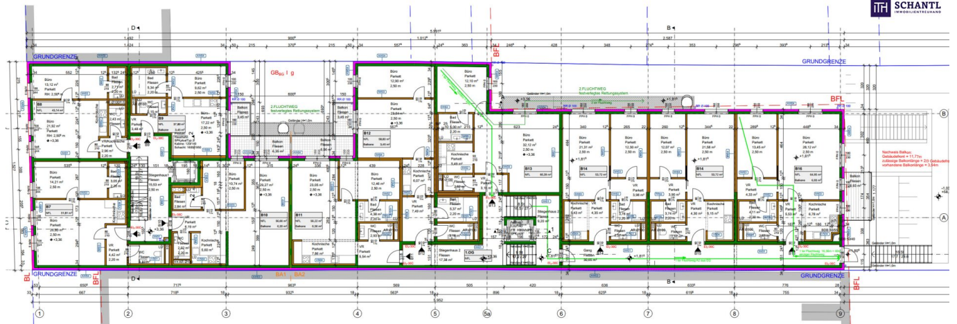
1. OBERGESCHOSS 1:100
