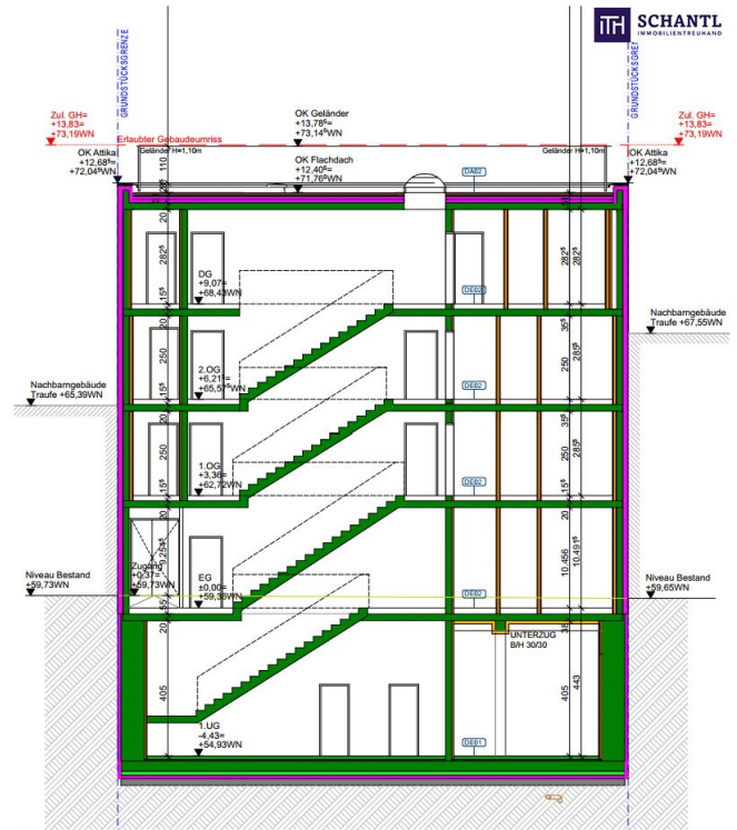
SCHNITT D-D 1:100
