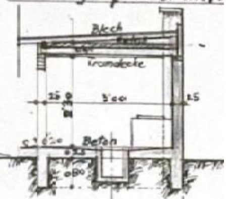
Garage querschnitt:
