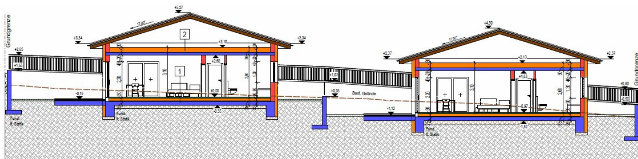
SCHNITT A-A
