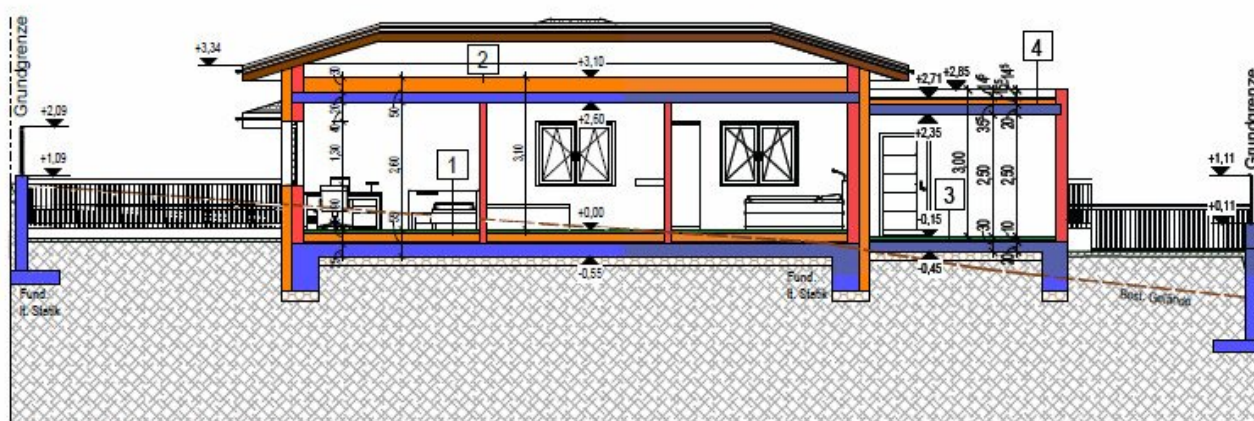
SCHNITT B-B
