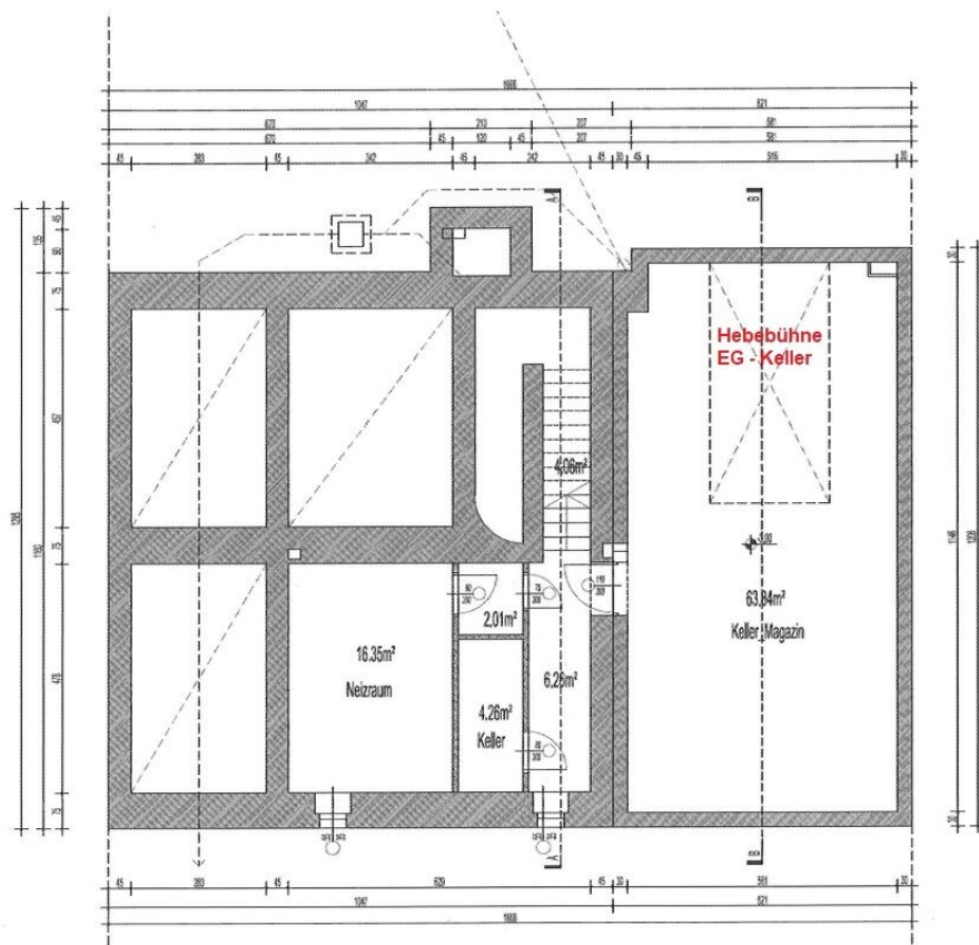
Kellergeschoss
