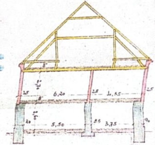
Schnitt A-B
