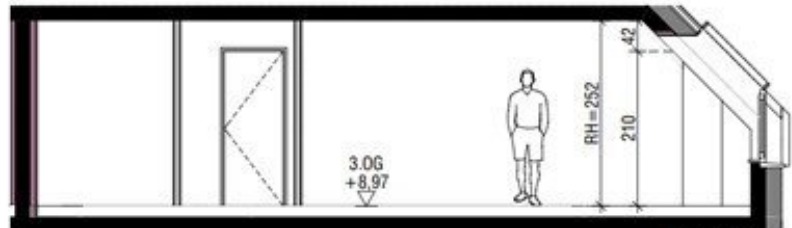
SCHNITT A
