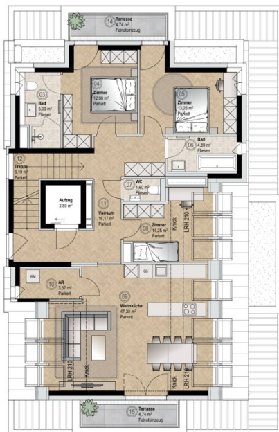
2. Dachgeschoss
