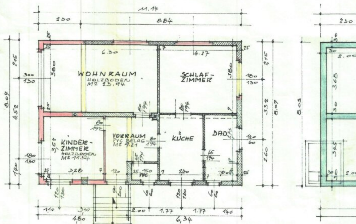
ERDGESCHOSS
