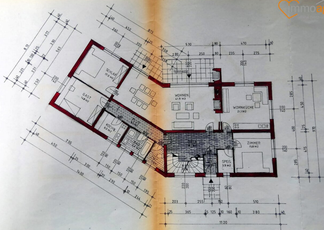
ERDGESCHOSS
