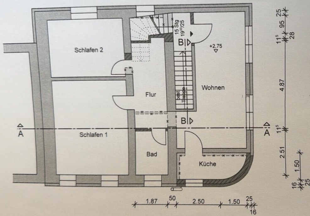
Grundriss Obergeschoss
