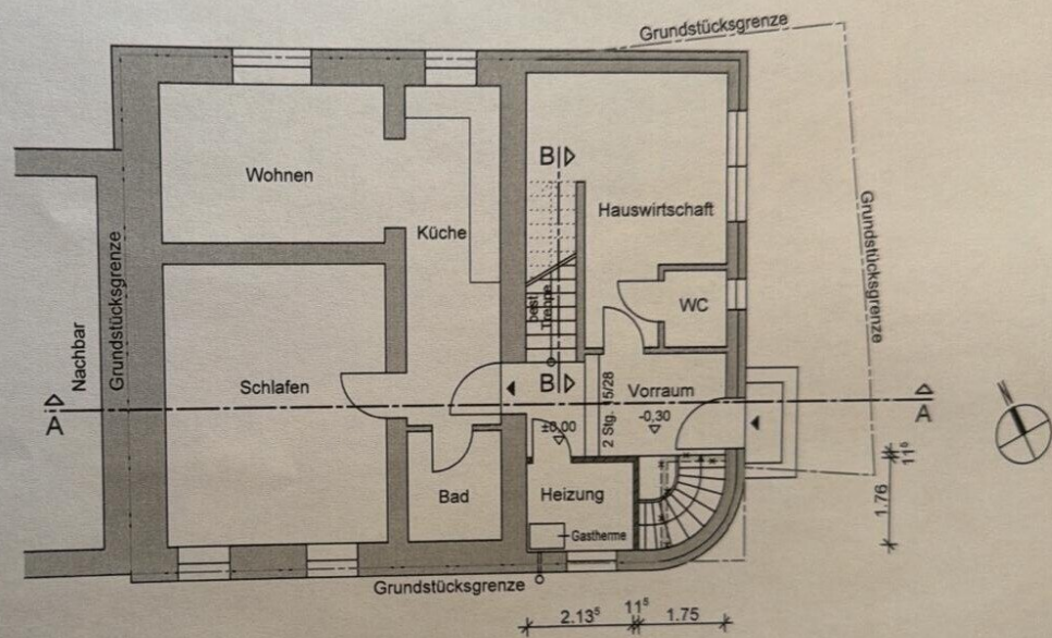
Grundriss Erdgeschoss
