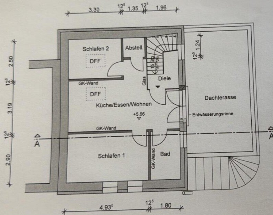
Grundriss Dachgeschoss
