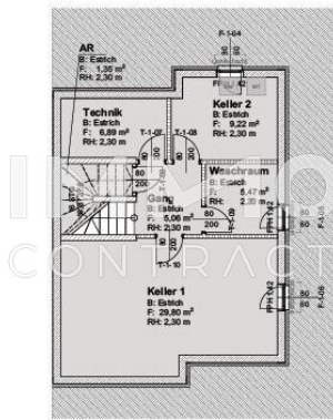
Reihenhausplan | RH 9, Kellergeschoss
