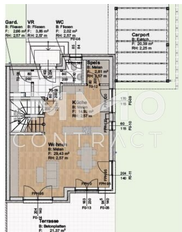
Reihenhausplan | RH 9, Erdgeschoss
