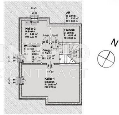
Reihenhausplan I RH 11, Kellergeschoss
