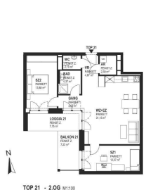
TOP 21 - 2.OG M1/100
