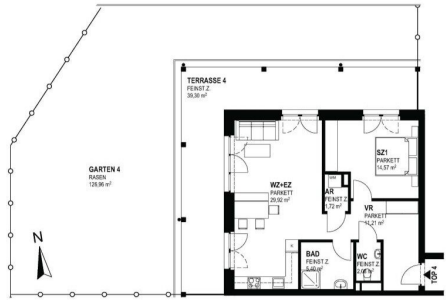
TOP 4 - EG M1:100
