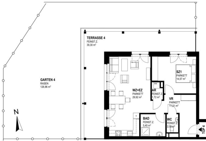
TOP 4 - EG M1:100
