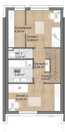
1. Obergeschoss Raumhöhe 2,53 m
