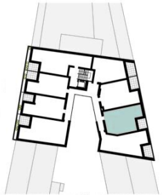
ORIENTIERUNGSPLAN | +1 OBERGESCHOSS
