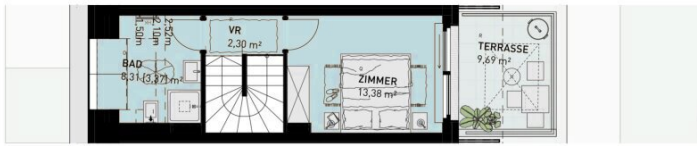
+2 DACHGESCHOSS
