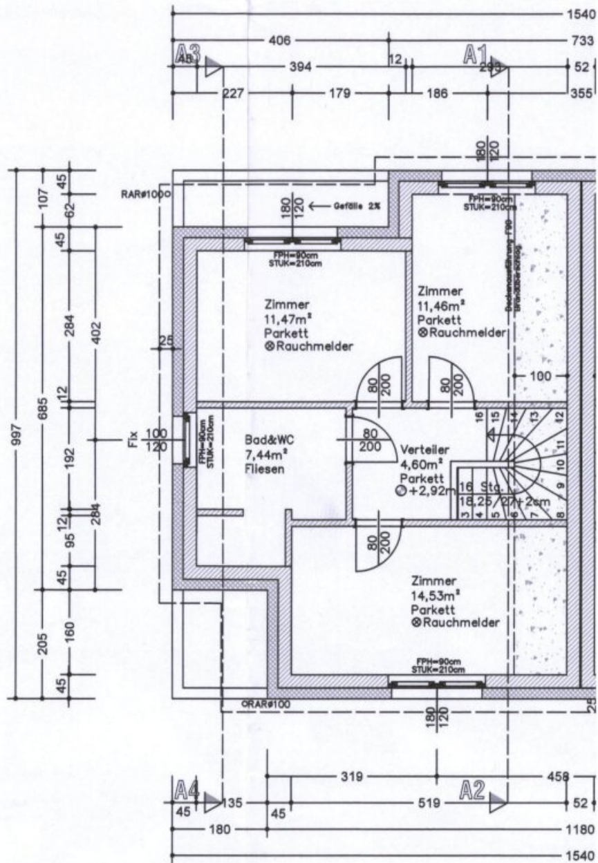
Grundriss Obergeschoss
