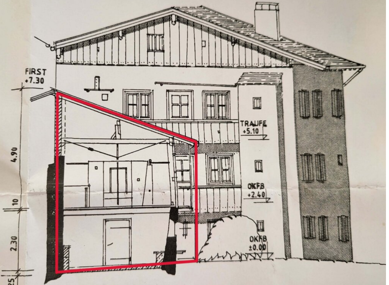
SCHNITT A-A
