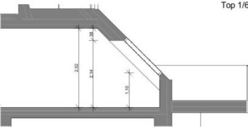
Schnitt 1/69 B
