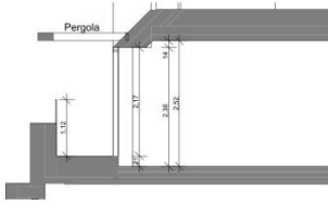
Schnitt 1/72 A
