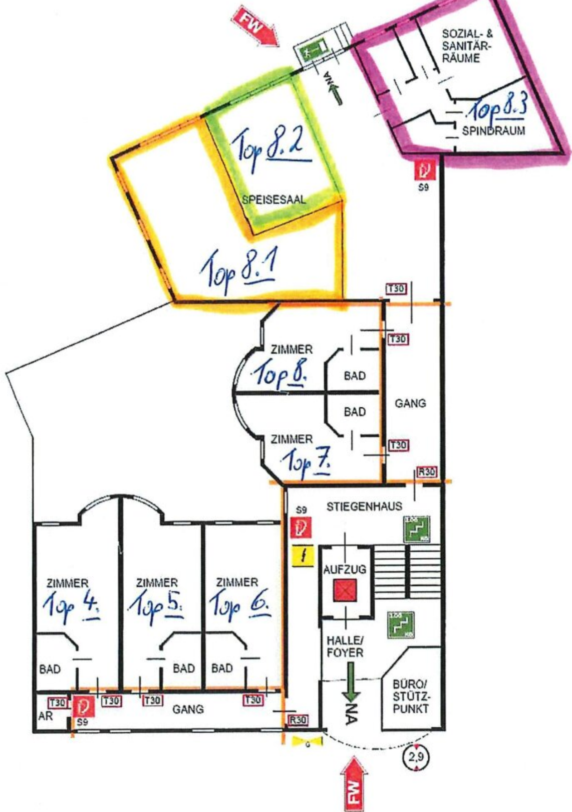
ERDGESCHOSS
