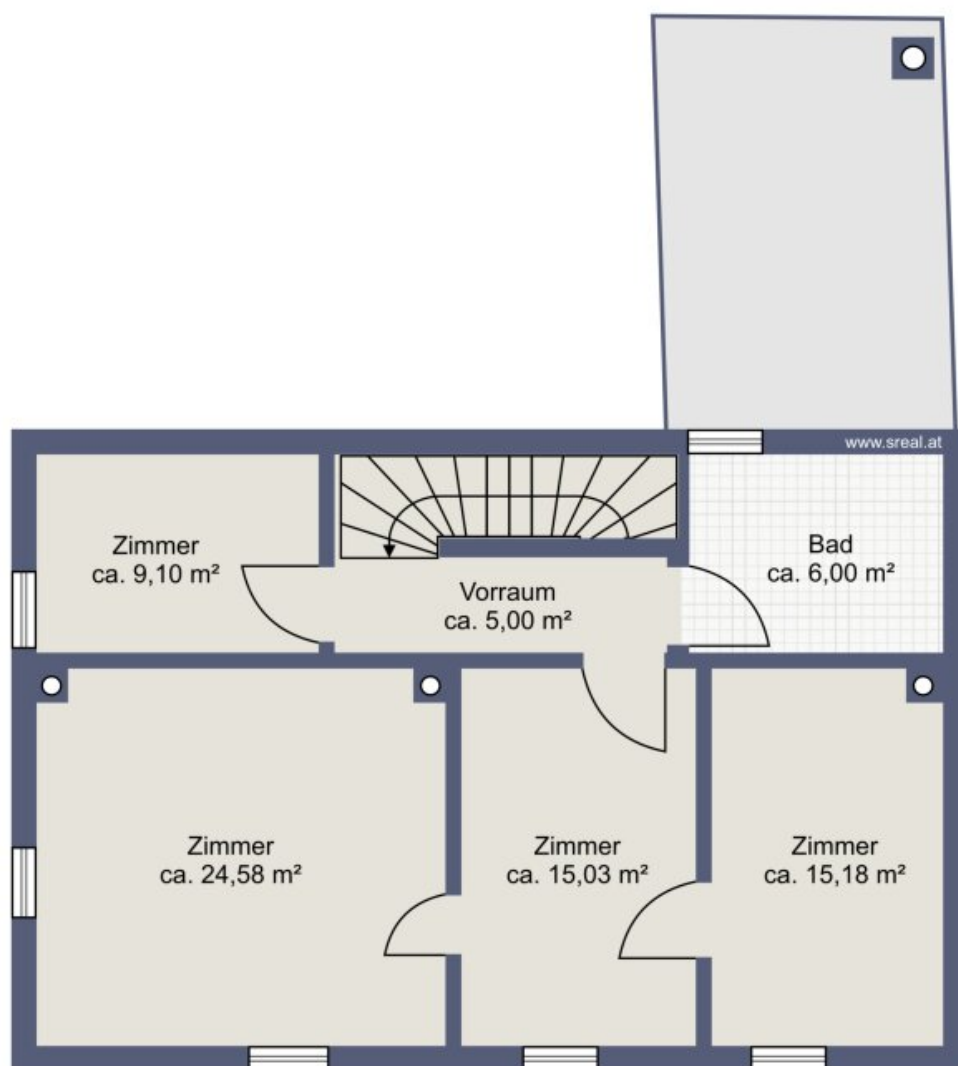
Skizze Dachgeschoss
