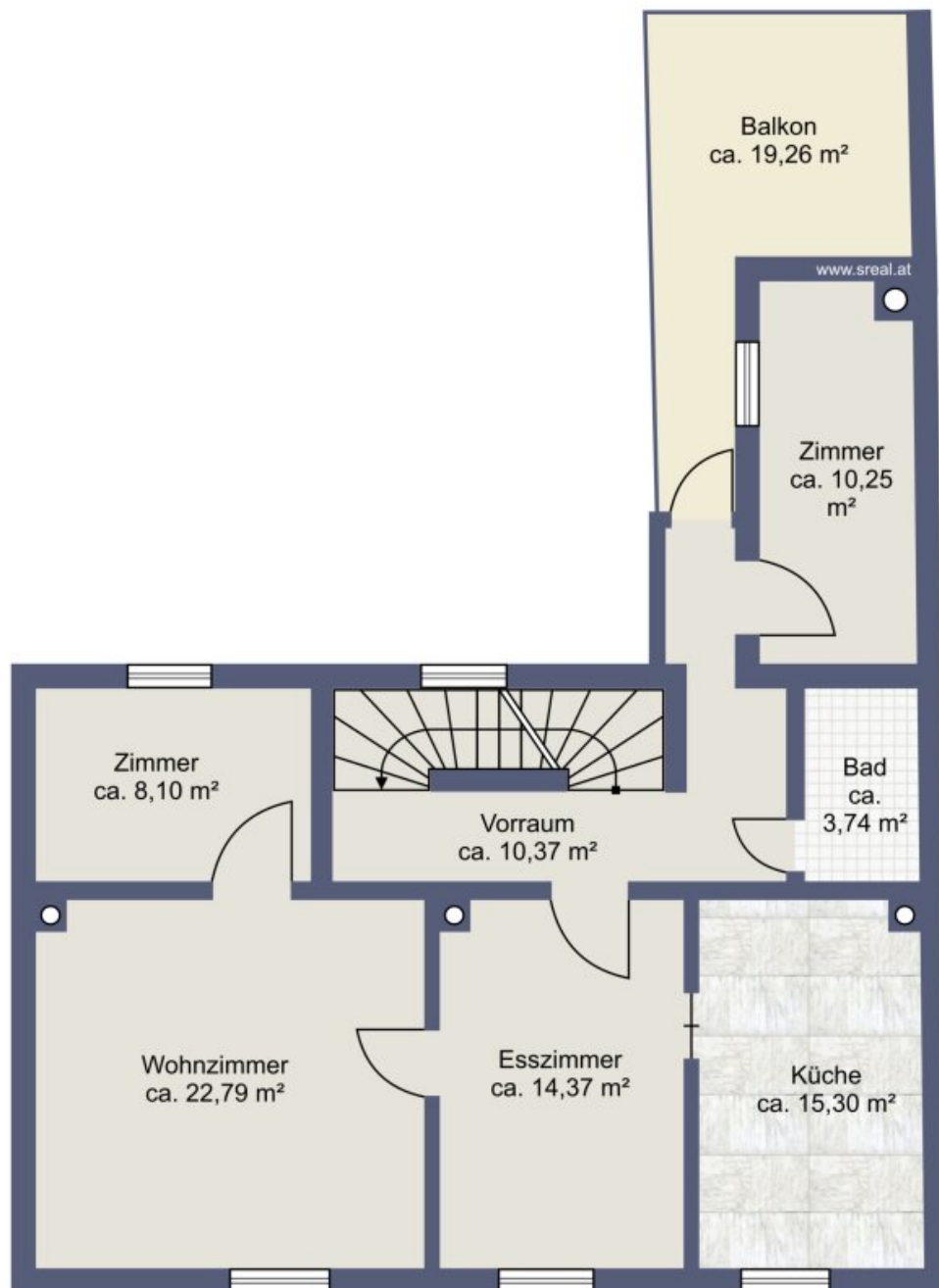
Skizze Obergeschoss
