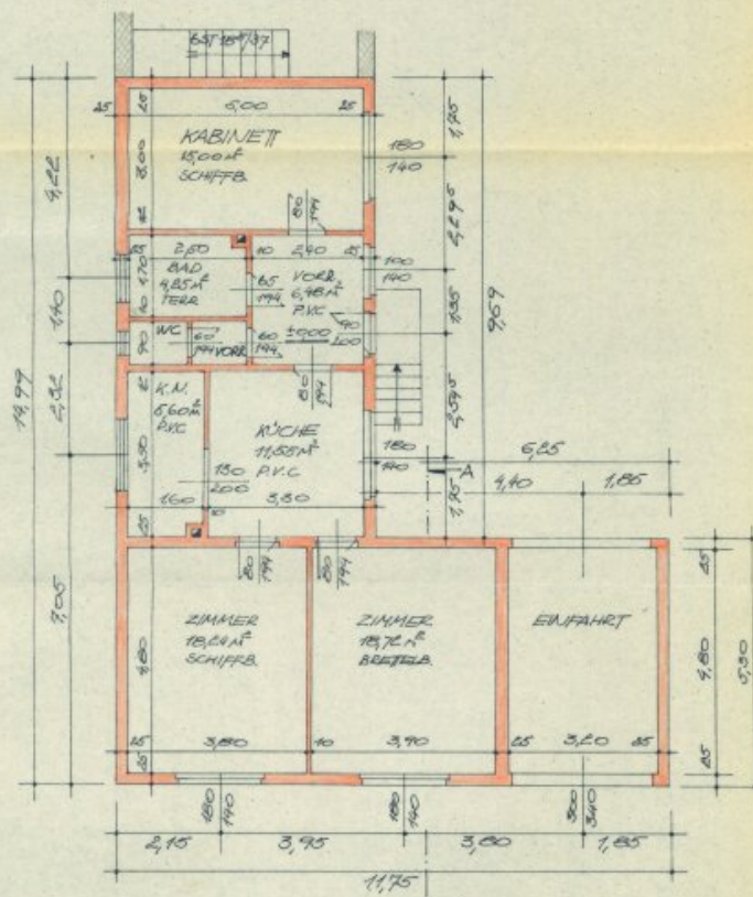
ERDGESCHOSS
