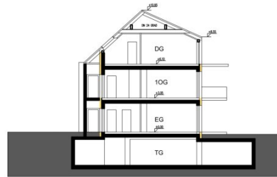
SCHNITT A
