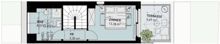
+2 DACHGESCHOSS
