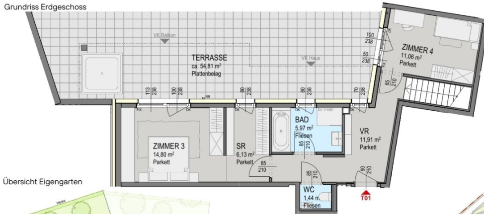
Grundriss Erdgeschoss
