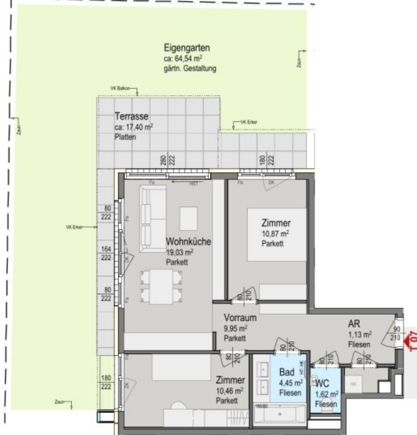
Grundriss Erdgeschoß
