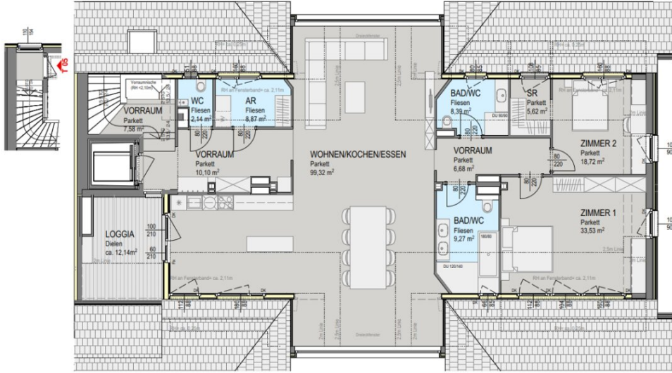
Grundriss Dachgeschoss
