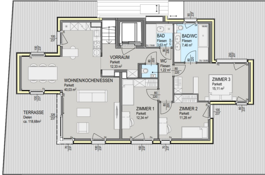
Grundriss Dachgeschoss
