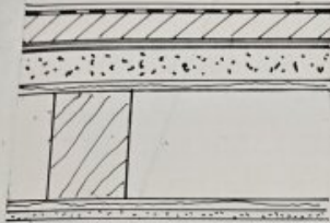
FUSSBODENKONSTR. BAD M. 1:10
