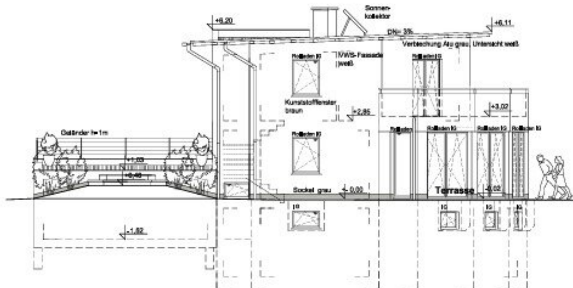
ANSICHT SÜDWEST
