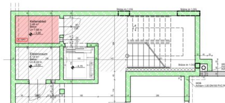
Planausschnitt KELLERGEHOSS - Abteil TOP 01 - OST Planstand = Ausführungsplan M: 1:100
