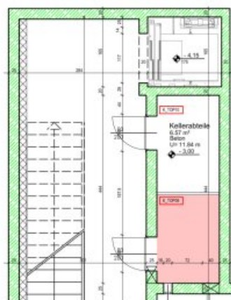
Planausschnitt KELLERGESCHOSS - Abteil TOP 09 - WEST Planstand = Ausführungsplan M: 1:100
