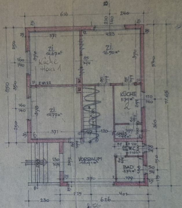
ERDGESCHOSS
