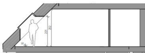
Schnitt 1-1
