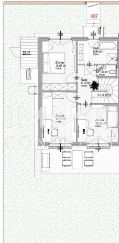
Obergeschoss
