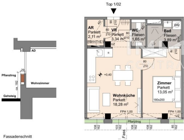
Fassadenschnitt
