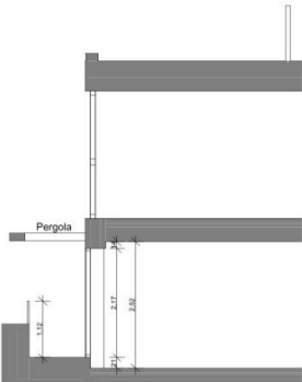
Schnitt 1/74 A
