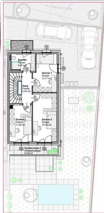
1. OG
