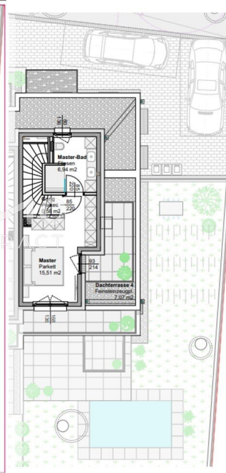
2. OG
