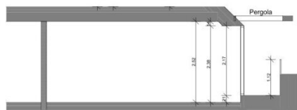
Schnitt 2/64 A
