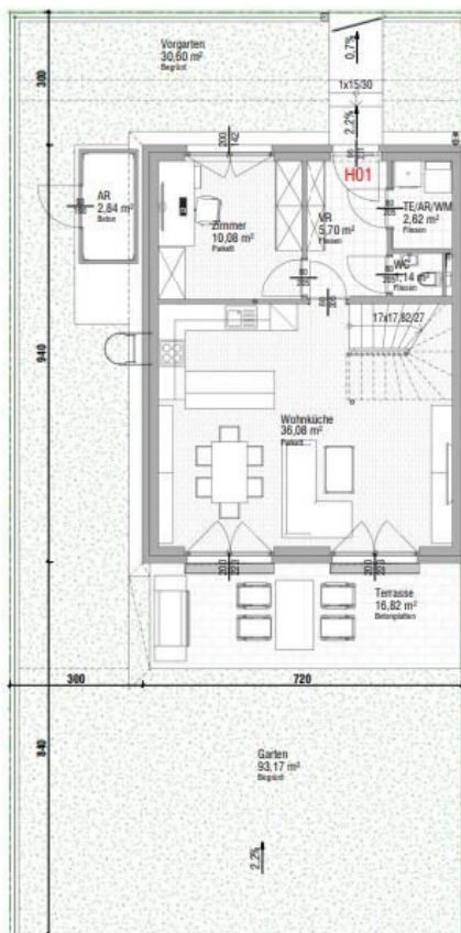
Erdgeschoss
