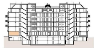
ERDGESCHOSS 2 ZIMMER
